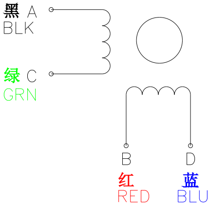
Wiring Diagram:
